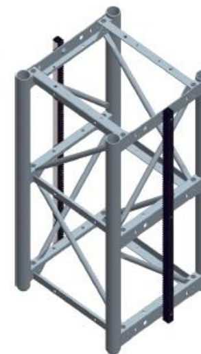
Ysc650A 标准节 Mast section
